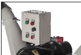
Steuerkasten
