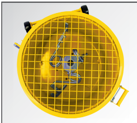
Das federnde 3-fach Rührwerk mischt das Material schnell & gründlich. Der Wandabstreifer verhindert Mischgutablagerungen an der Trommelwand.
