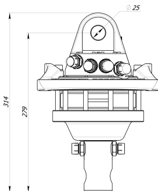
FHL 01B-A/B-60/25
