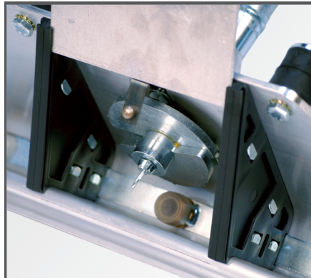
Variable Fliehkraft passend zur Patschenbreite und zum Setzmaß.
