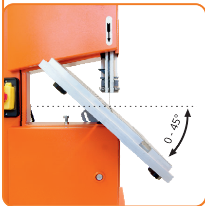
neigbarer Sägetisch 0° bis 45°
