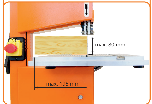
maximal zu sägende Werkstückhöhe und -breite
