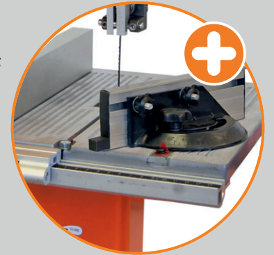
maximal zu sägende Werkstückhöhe und -breite
