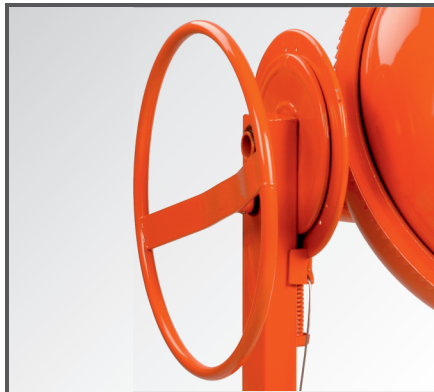
Großes Handrad mit leichtgängigem Schwenkgetriebe, Scheibenbremse & Fußbediening für das stufenlose Verstellen der Mischtrommel.
